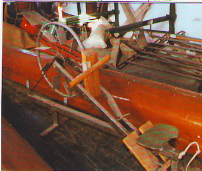
«Concept II» kakvog su izradili veslački djelatnici VK Croatije početkom 70-ih godina za svoje veslače a nešto kasnije koristile su ih generacije zagrebačkih veslača.
